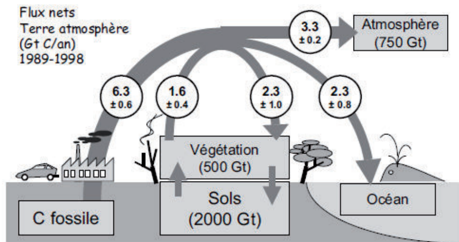
Figure 2 : Cycle global du carbone. Les échanges entre les réservoirs et les bilans sont exprimés en milliards de tonnes (ou giga tonnes) de carbone par an.
